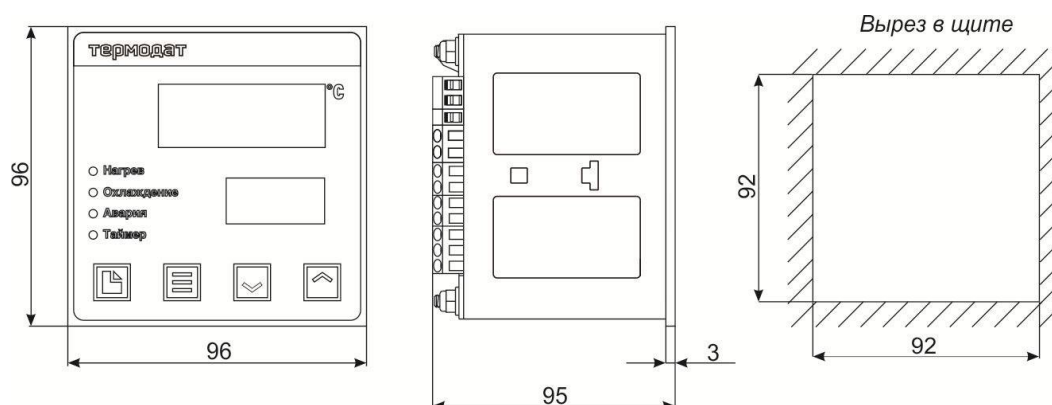
Рисунок 17 – Габаритные размеры прибора Термодат-12К6-D4/.....
