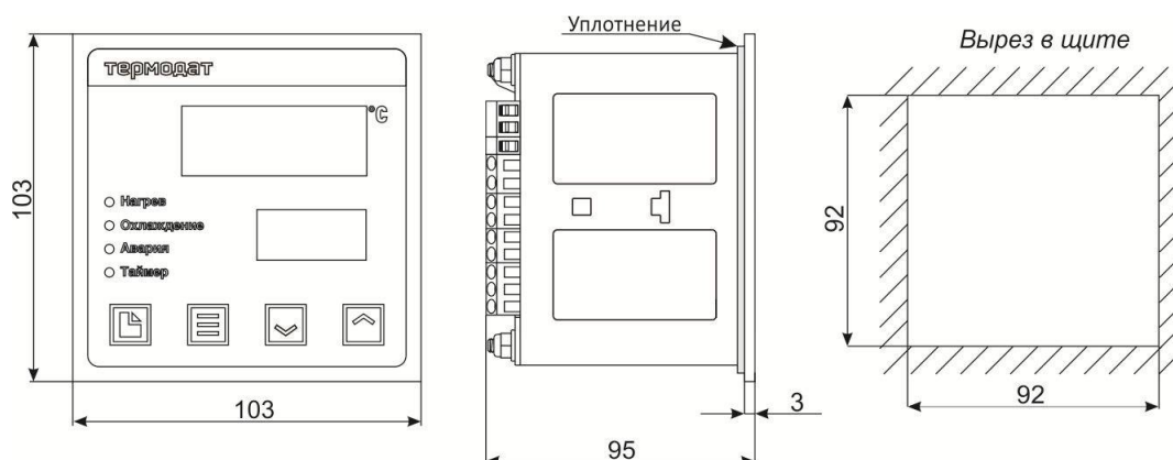
Рисунок 18 – Габаритные размеры прибора Термодат-12К6-D4/...../ IP67pp
