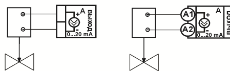
Подключение задвижки с электроприводом
