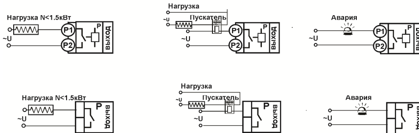
Подключение нагрузки менее 1,5 кВт
