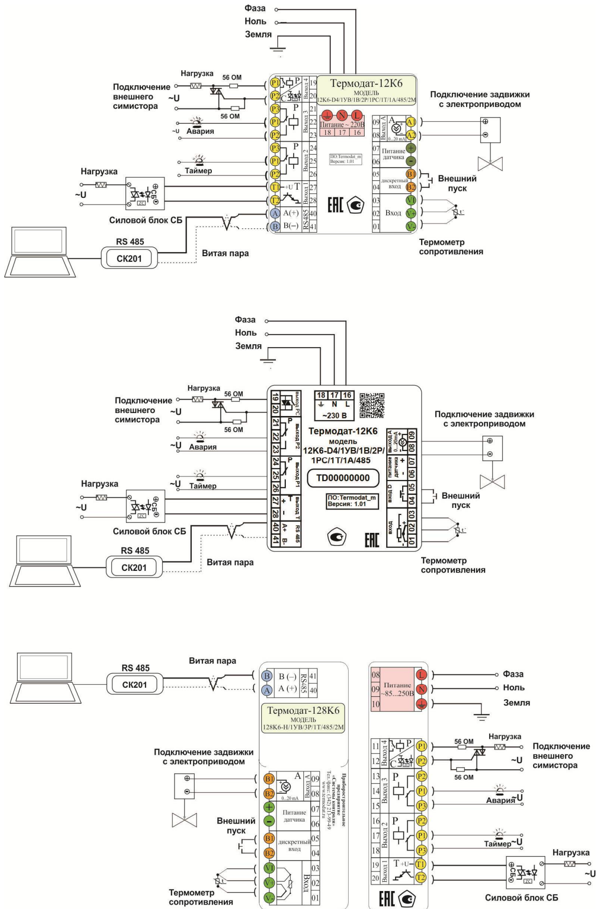
Рисунок 16 – Типовая схема подключения прибора
