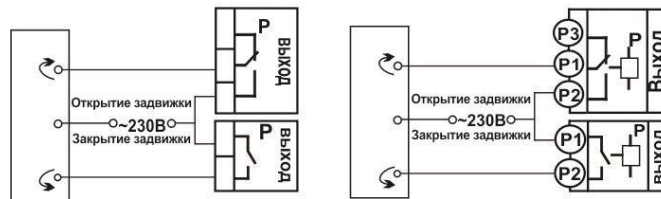
Подключение электрозадвижки
