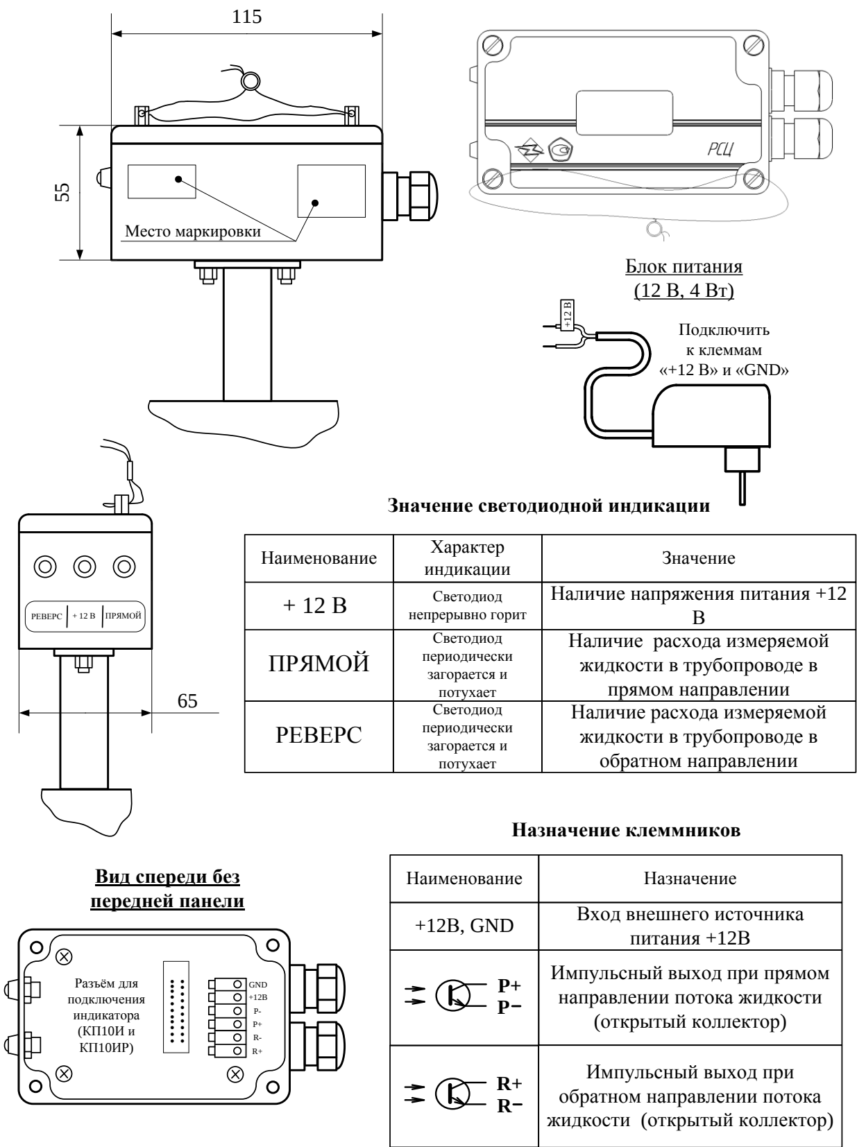
Рисунок Г.4 - Блок измерительный с креплением к ГП исполнение «Ф00» (КП10, КП10ИР)
