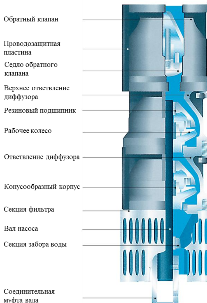
Рисунок 14. Структура насосной части погружного агрегата насосного SJ
